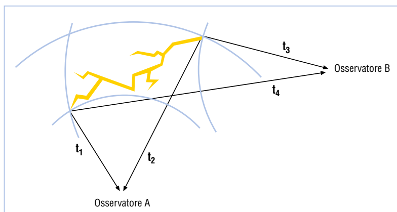
Figura 3: Rappresentazione schematica del perché uno stesso fulmine produce un tuono sentito in maniera diversa da due osservatori. Grazie all'alta velocità di propagazione della luce, l'osservatore A e l'osservatore B vedranno il fulmine nello stesso istante t_0 ma l'osservatore A sentirà il tuono nell'intervallo compreso tra il tempo t_1 e il tempo t_2 , contati a partire da quando il fulmine è stato visto; l'osservatore B, al contrario, lo sentirà tra il tempo t_3 e il tempo t_4 . Poiché i quattro tempi differiscono, diversa sarà anche la durata del tuono per A e B.
