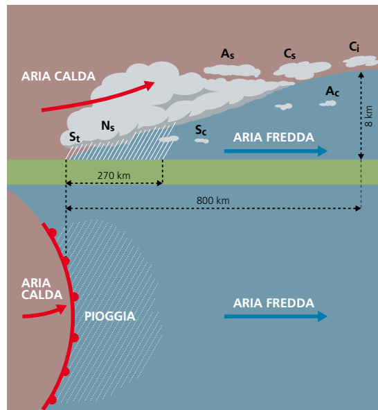
Fig. 20 Sezione verticale di un sistema frontale (riquadro B della fig. 19)
