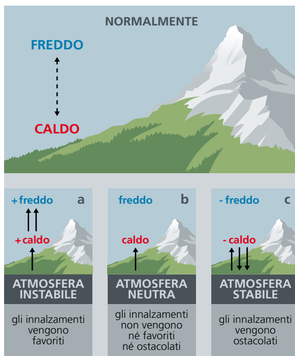
Fig. 27 Atmosfera instabile, neutra e stabile
