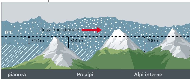
Dipendenza del limite della nevica: fig. 33 – da eventuali inversioni termiche; fig. 34 – dall'ampiezza della valle; fig. 35 – dalla posizione geografica
