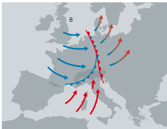
Fig. 44 Schema di un sistema frontale sulle Alpi
