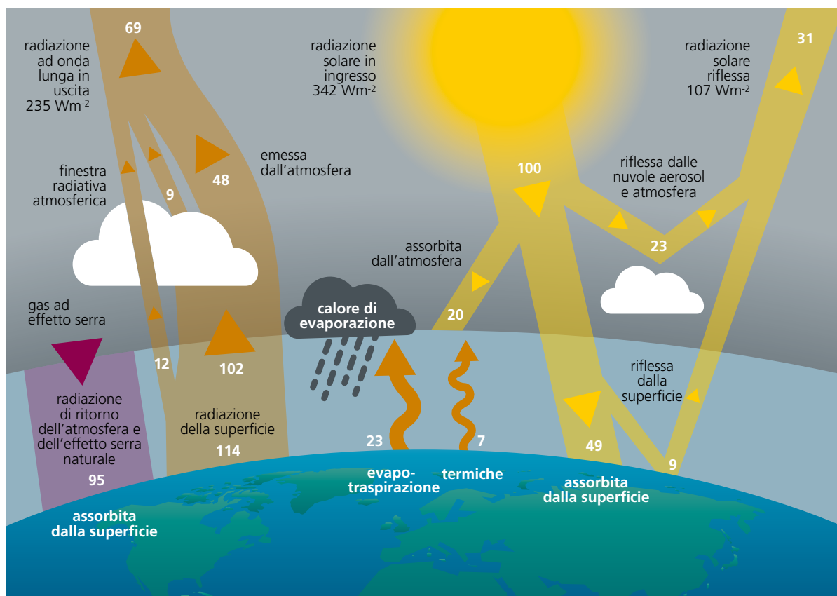
Fig. 1 Schema semplificato del bilancio radiativo terrestre
