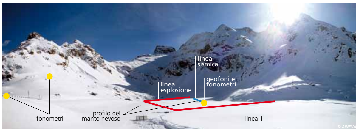
Fig. 4 - Vista del campo prove il giorno 31 marzo 2010. Sono indicati: la linea di tiro (in rosso), la traccia dello stendimento geosismico (in blu) e i differenti punti monitoraggio.
