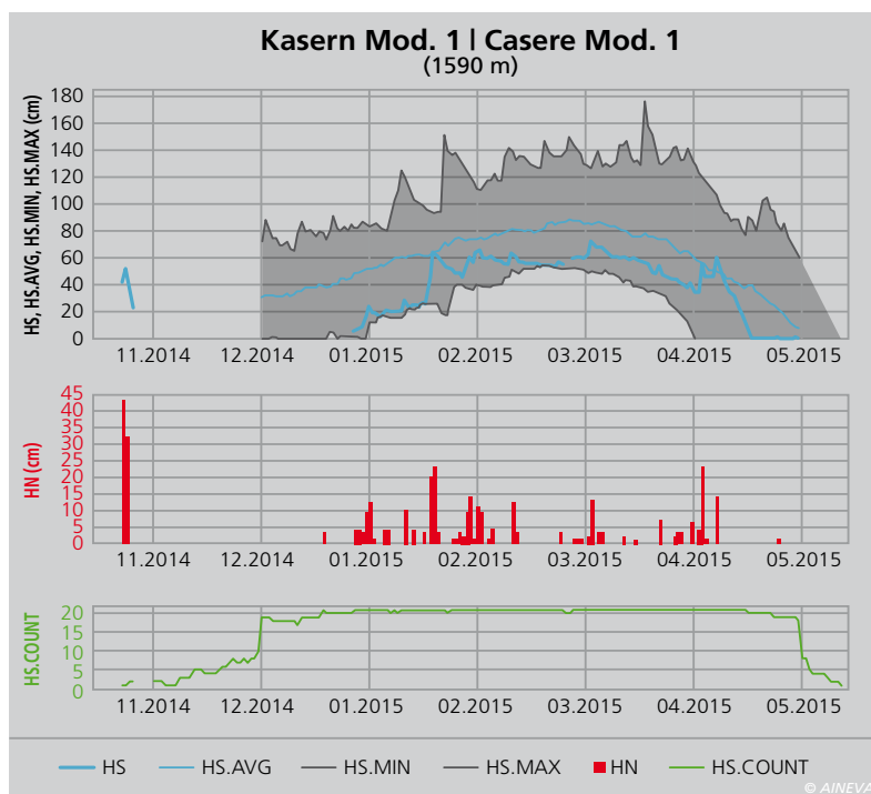
Fig. 27 - Sopra l'altezza neve, sotto la neve fresca misurata dall'osservatrice a Casere in Valle Aurina. Spiegazione: nel riquadro superiore i bordi della fascia grigia rappresentano il minimo e il massimo storico misurato nel lungo periodo (inverno 94/95 fino 2013/14). La linea blu sottile raffigura la misura media e quella più grossa l'andamento della neve al suolo nell'inverno 2014/15. Nel riquadro inferiore le linee rosse verticali raffigurano la neve fresca misurata giornalmente durante l'inverno.
