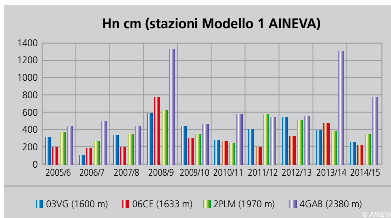
Fig. 44 - I valori cumulati stagionali delle precipitazioni nevose degli ultimi 10 anni in 4 stazioni di Modello 1 AINEVA.
