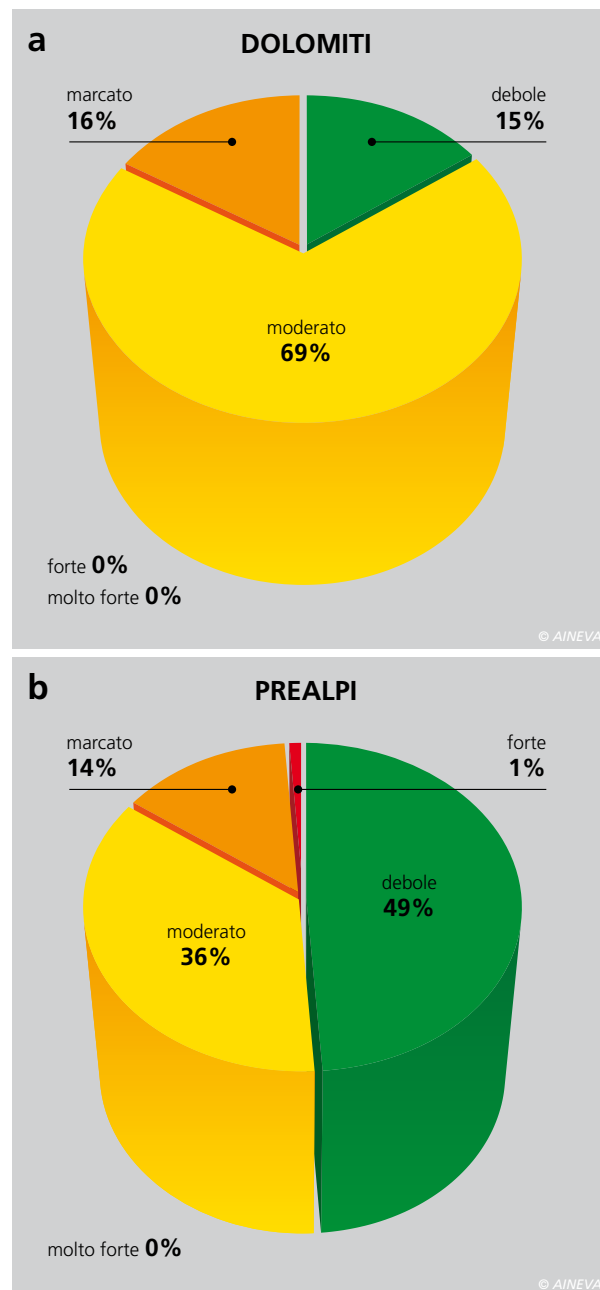
Fig. 6 - Distribuzione del pericolo di valanghe sul territorio durante la stagione invernale 2014/2015.
