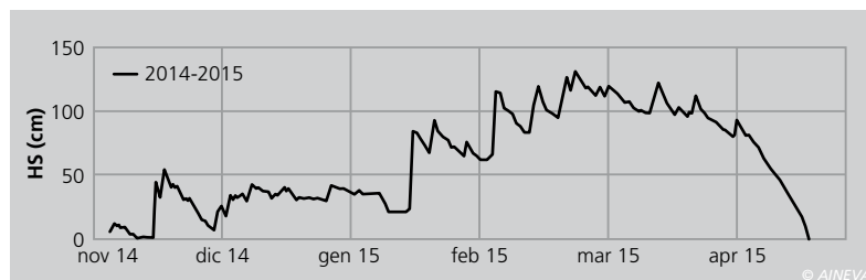
Fig. 13 - Altezza neve al suolo di Passo Tonale (1880 m s.l.m.) nel settore occidentale del Trentino.
