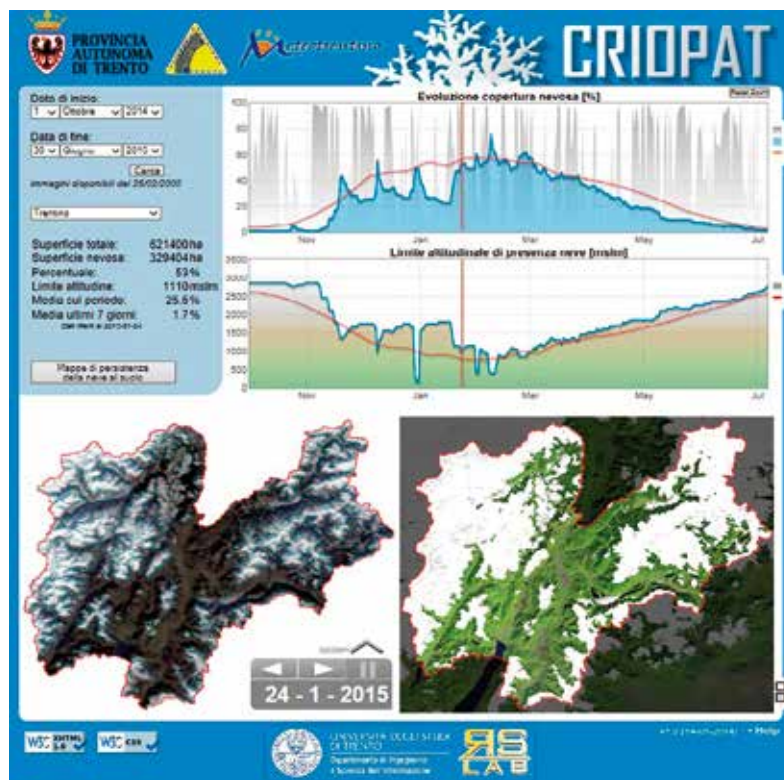
Fig. 12 - CrioPat: andamento stagionale della copertura nevosa del Trentino con immagini e dati del 24 gennaio 2015.
