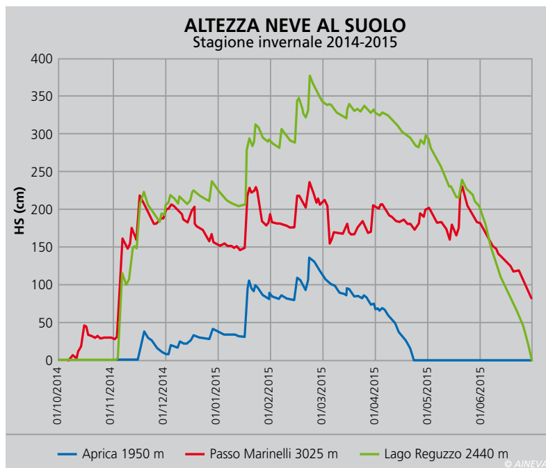
Fig. 32 - Evoluzione dell'altezza del manto nevoso al suolo in tre stazioni rappresentative per quota e settore di appartenenza.
