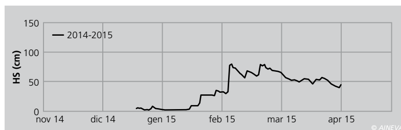
Fig. 15 - Altezza neve in loc. Vason del Bondone (1670 m s.l.m.) nel settore centrale del Trentino.
