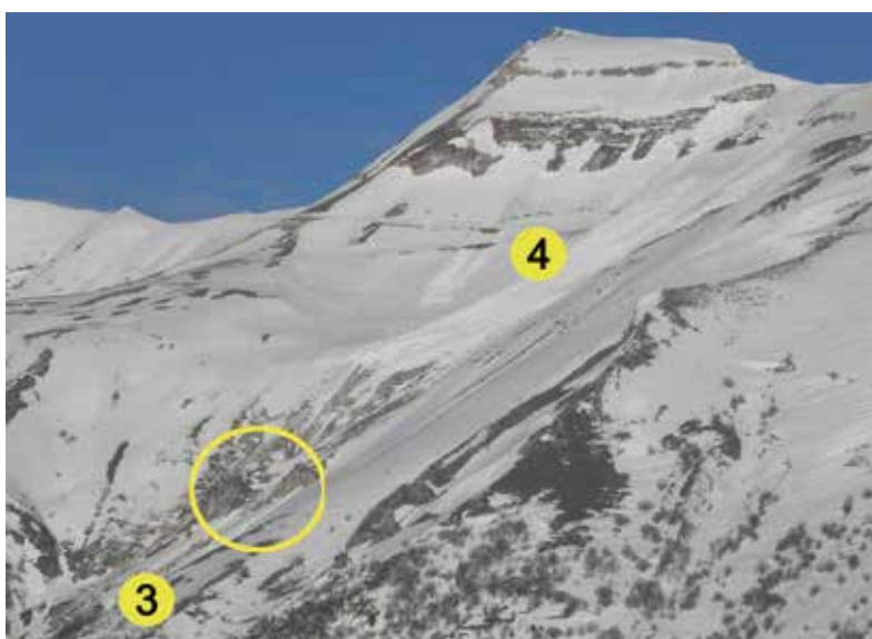
Fig. 58 - Area di distacco del sito valanghivo n.3 e n.4.
