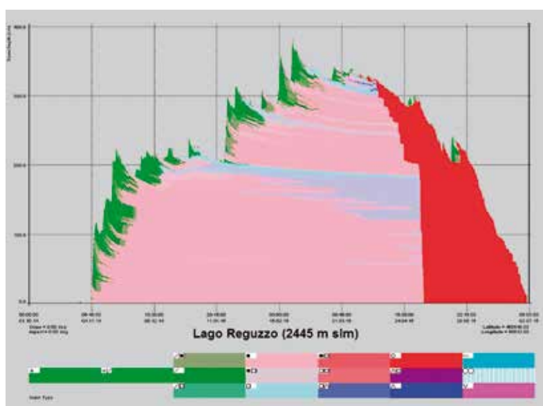
Fig. 40 - Evoluzione cristallografica stagionale del manto nevoso, presso la stazione di Lago Reguzzo (Orobie), simulata tramite software SNOWPACK.
