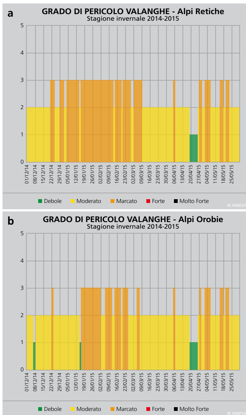
Fig. 39 - Il Pericolo Valanghe ha visto prevalere un indice 3 MARCATO sui settori retici e Adamello., 2 MODERATO sui settori orobici e prealpini.
