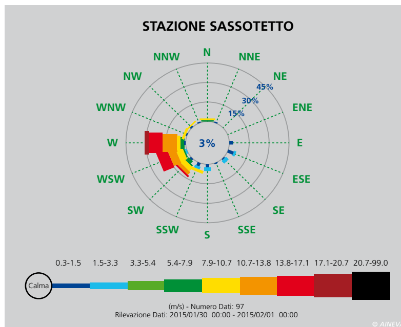
Fig. 54 - Rosa dei venti per le giornate di venerdì 30 e sabato 31 gennaio 2015 della stazione nivometrica automatica di Sassotetto (versante orientale dei Sibillini).
