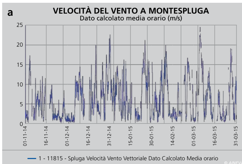
Fig. 34 - a) rappresentazione grafica della velocità del vento registrata presso la stazione di Montespluga; b e c) tipici esempi di eventi nivometeorologici caratterizzati dal presenza di stau sul versante nordalpino e di föhn sul versante prospiciente la pianura Padana 2 marzo e 22 ottobre.
