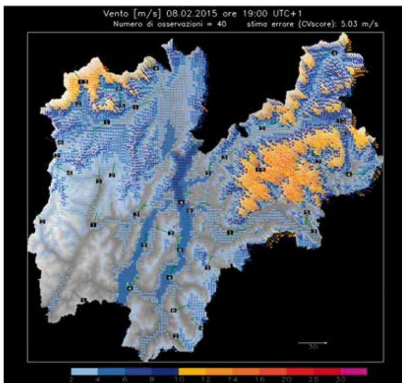
Fig. 17 - Mappa del vento sul Trentino dell'8 febbraio 2015.
