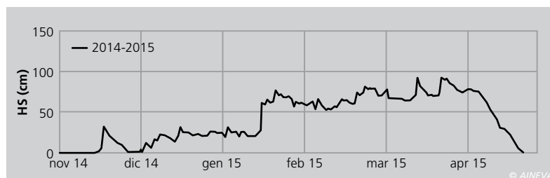
Fig. 14 - Altezza neve Passo Rolle (2012 m s.l.m.) nel settore orientale del Trentino.
