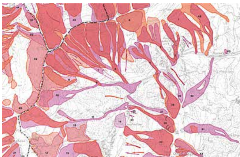
Fig. 57 - Particolare della CLPV per il comune di Montemonaco (Sibillini sudorientali).
