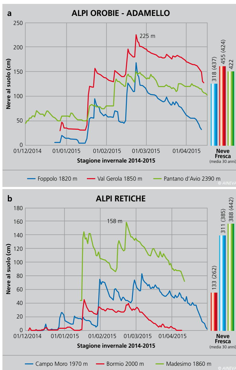
Fig. 33 - Cumuli di neve fresca nella stagione invernale 2014-2015, registrati presso le stazioni tradizionali nivometeorologiche lombarde.
