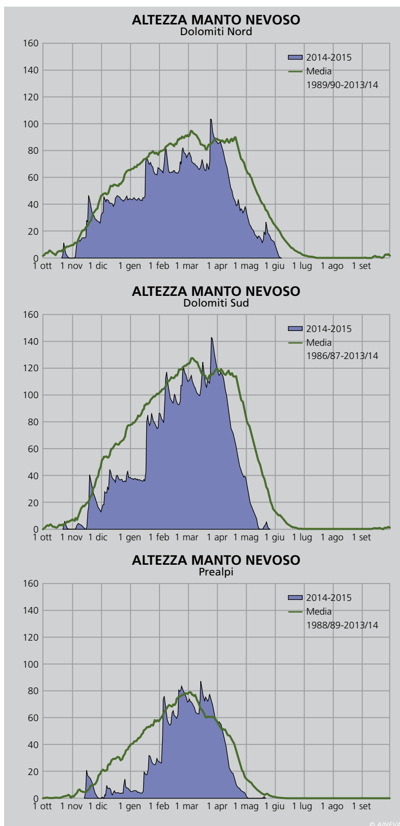
Fig. 5 - Altezza del manto nevoso nella stagione invernale 2014/15 rispetto alla media 1989/90-2013/2014 suddivisa per aree.
