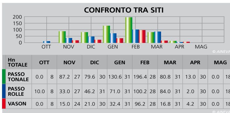
Fig. 18 - Confronto delle accumulate mensili di neve fresca (HN) tra stazioni indicative dei settori occidentale, orientale e centrale del Trentino. In tabella i valori numerici mensili di HN in centimetri con i giorni di osservazione mensile in apice.
