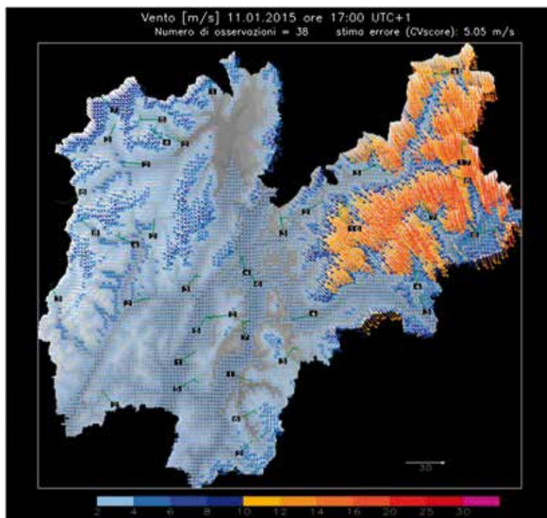
Fig. 16 - Mappa del vento sul Trentino dell'11 gennaio 2015.
