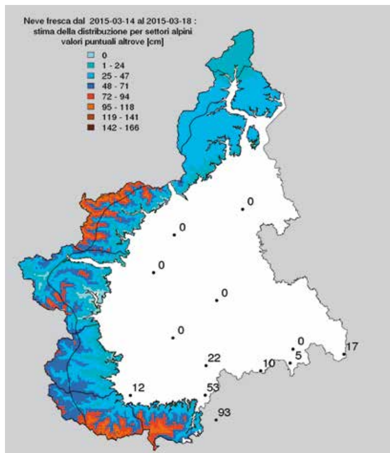
Fig. 50 - Cumulata nevicate dal 14 al 18 marzo 2015.
