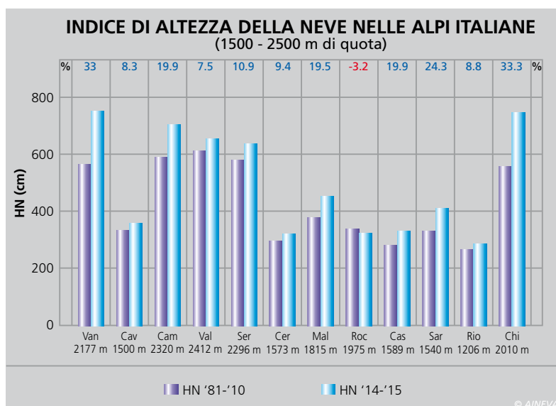
Fig. 46 - Neve fresca cumulata da novembre a maggio nella stagione 2014-2015 (in azzurro) a confronto con la media trentennale '81-'10 (in blu).
