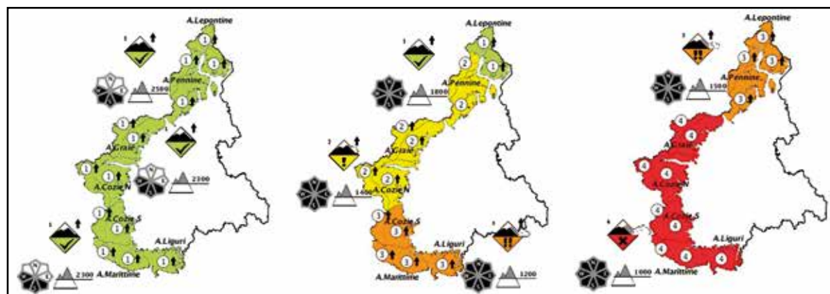
Fig. 51 - Grado del pericolo valanghe del 14, 15 e 16 marzo 2015.
