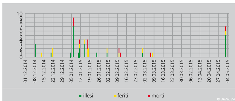
Fig. 29 - Incidenti da valanga inverno 2014/15.
