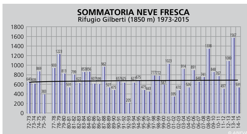
Fig. 1 - Sommatoria di neve fresca alla stazione Rifugio Gilberti (1850 m) dal 1973 al 2015.
