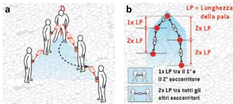
Fig. 1 - Disposizione e distanza dei soccorritori.
